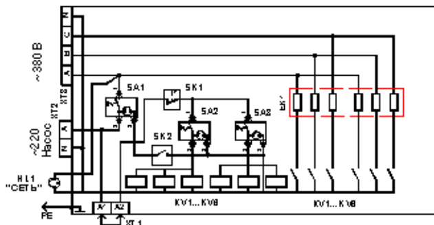
Рис. 10 ЭВПМ-12(бреле-6ТЭН). Схема электрическая принципиальная.
