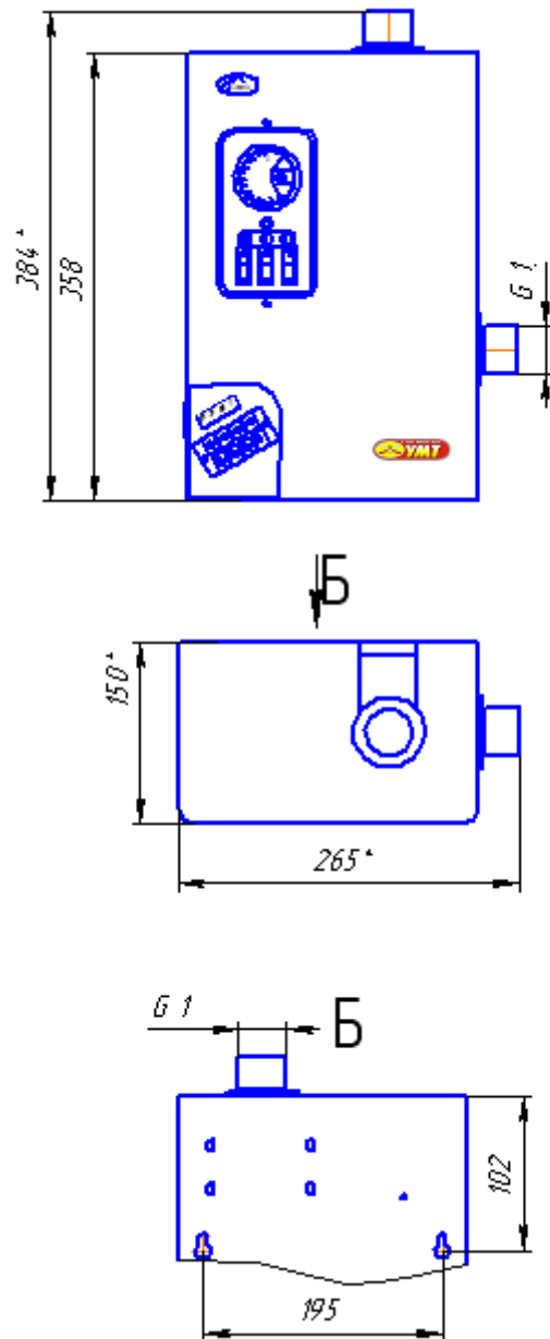
Рисунок 1 – Электронагреватель ЭВПМ-3...12
