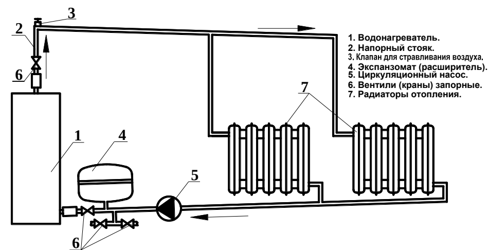
Рис. 11 Упрощенная схема включения ЭВПМ-3...12 в циркуляционную отопительную систему.
