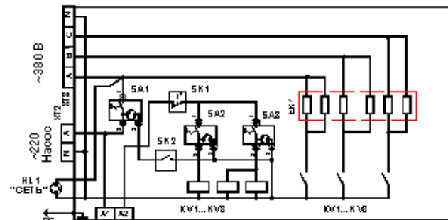
Рис. 9 ЭВПМ-9...12(Зреле-6ТЭН). Схема электрическая принципиальная.
