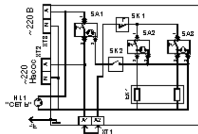
Рис. 7 ЭВПМ-3 Схема электрическая принципиальная.
